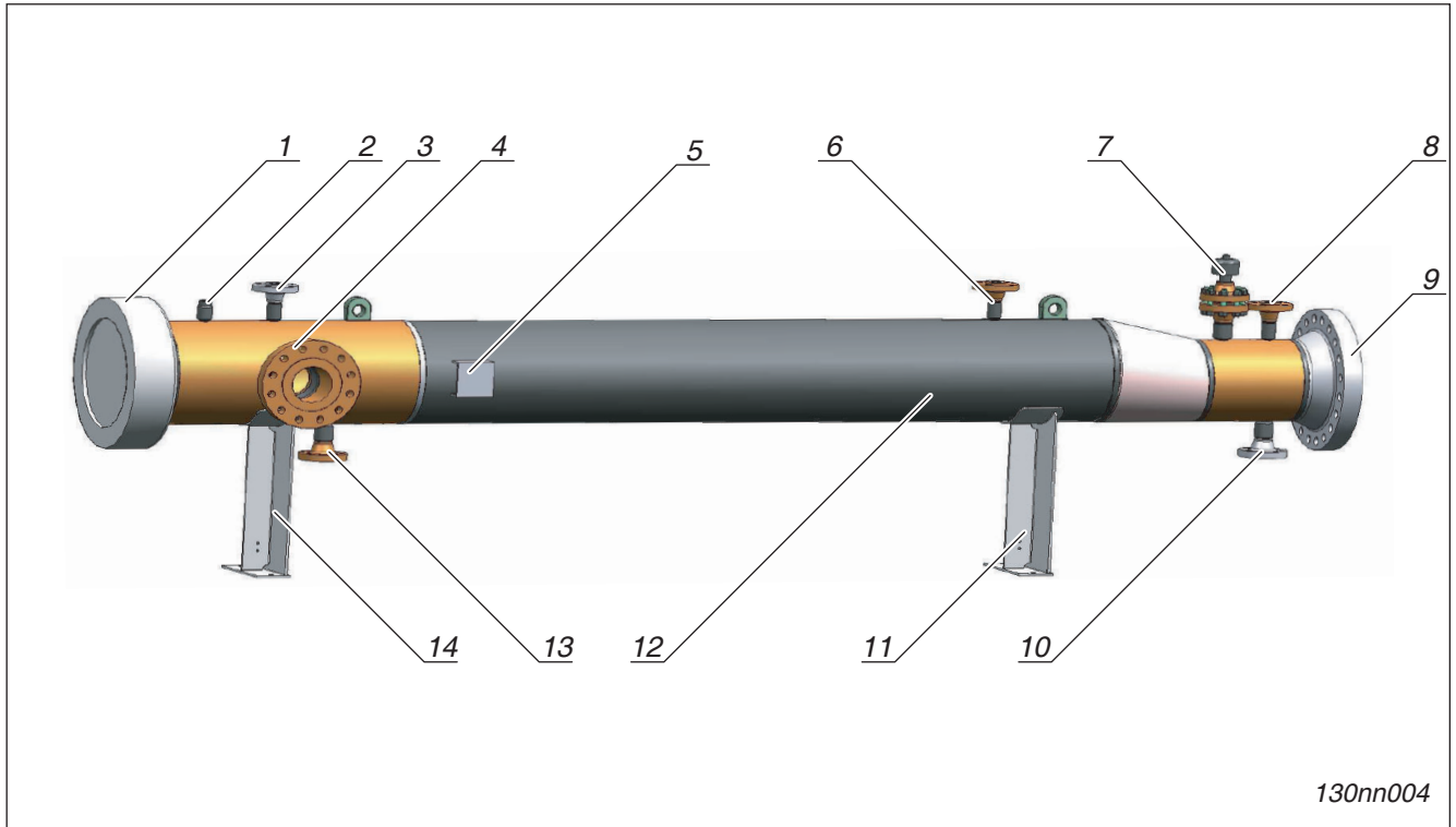
Fig. 3-1 Molchschleuse
